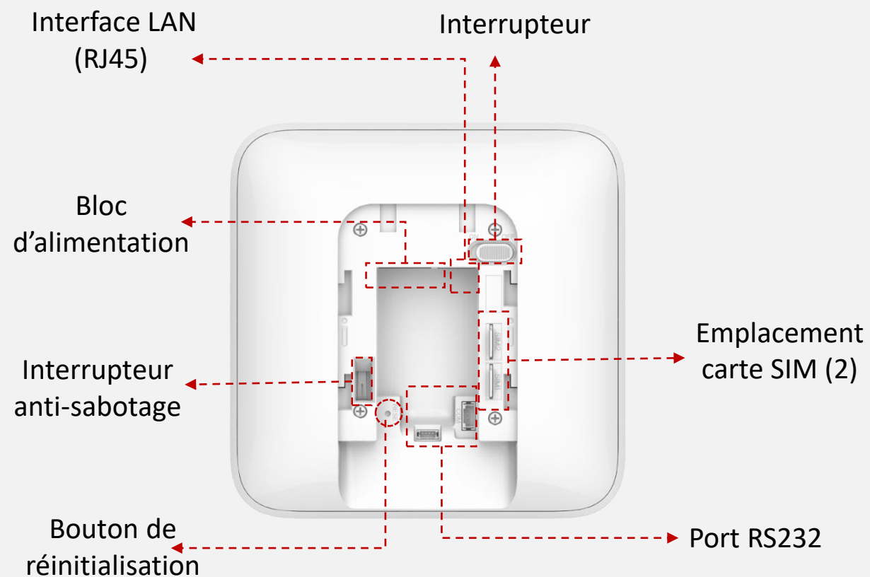
• Face arrière de AX PRO
